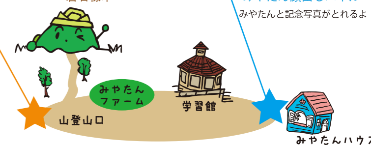
～岩石標本～
